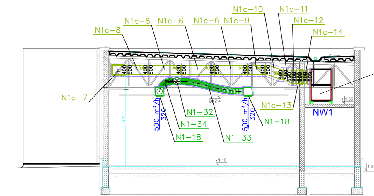
PRZEKRÓJ C-C
