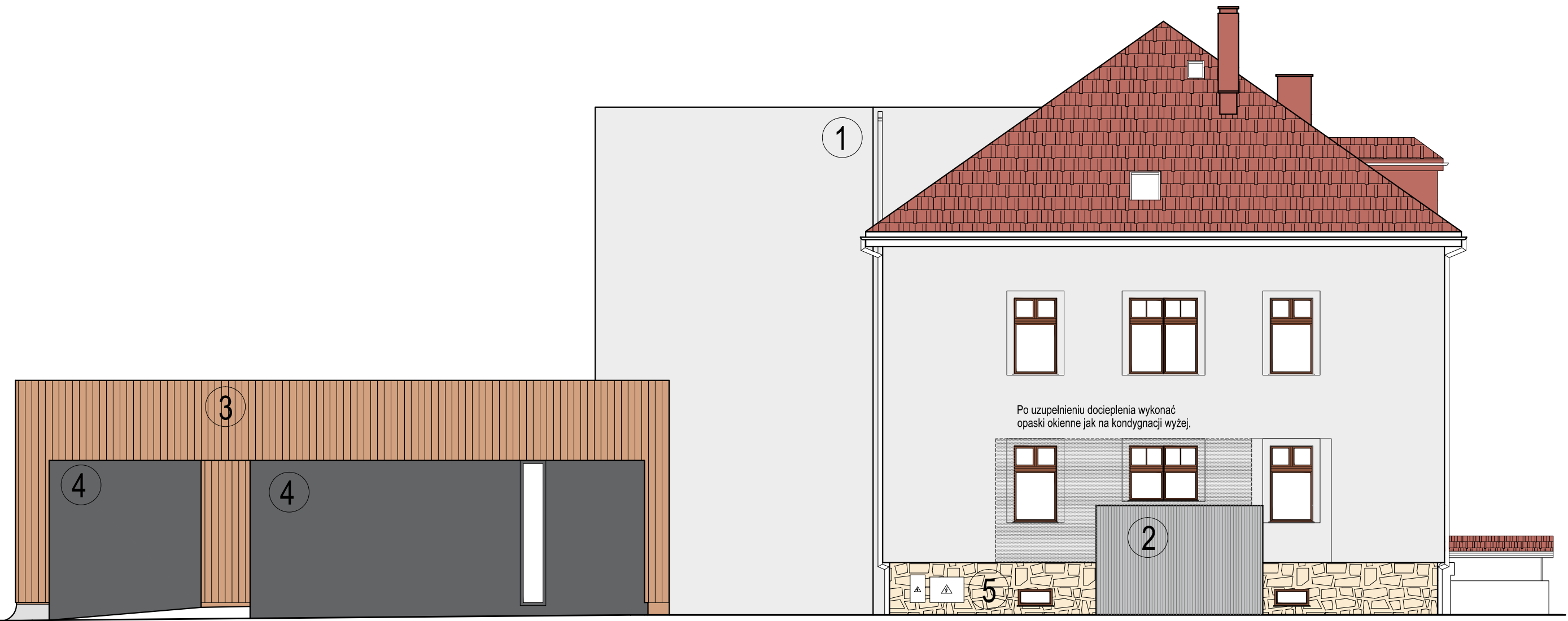
ELEWACJA POŁUDNIOWO-WSCHODNIA
